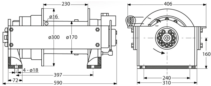
Dimensions in mm / Dimensiones en mm
